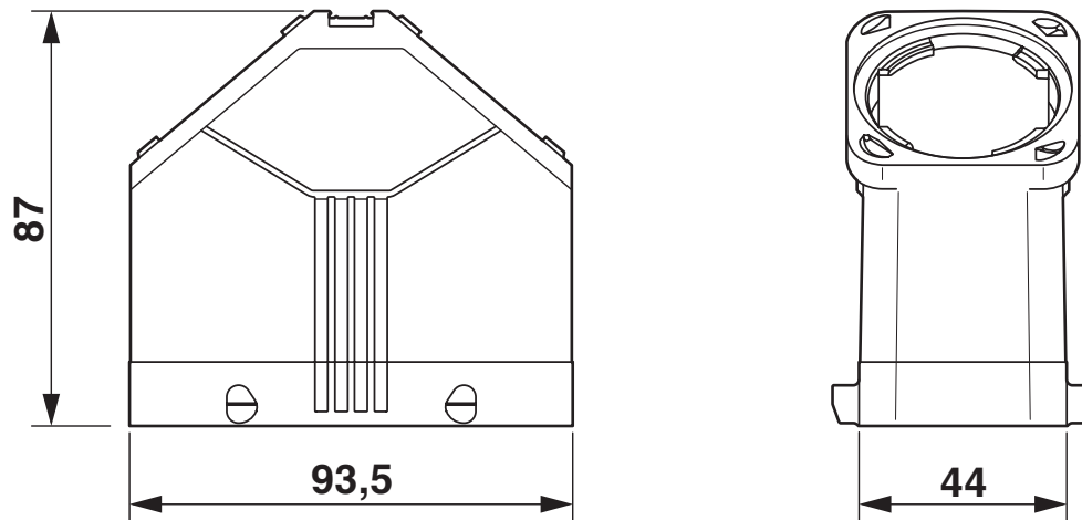
Maßzeichnung
