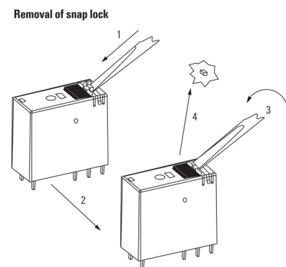
Detailzeichnung Entfernen der Rastsperrre der Prüftaste
