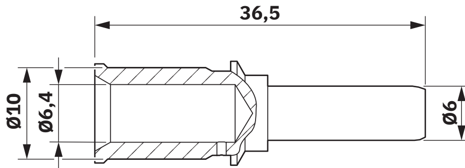
Dessin coté
