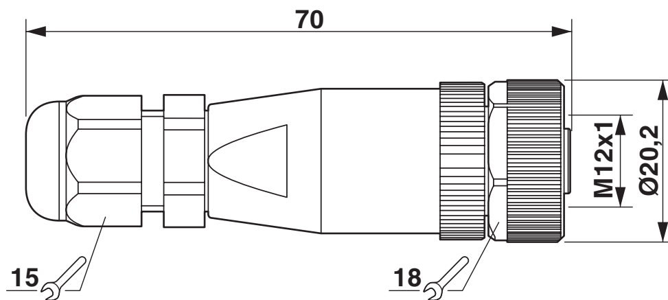
Maßzeichnung
