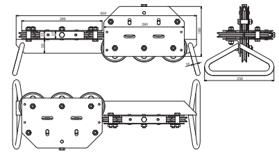
Maßbild DRG 10RO 7.10 HG STGALZN
