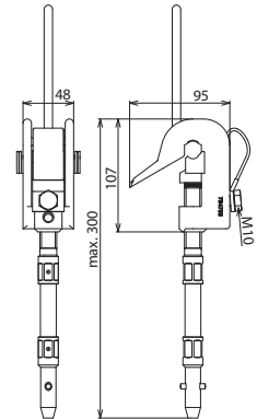
Maßbild FEK 4 15 TS FSQL
