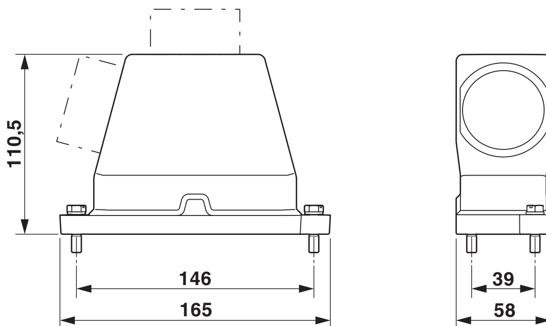
Dessin coté
