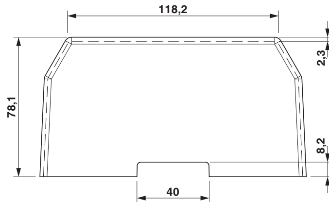
Dessin coté
