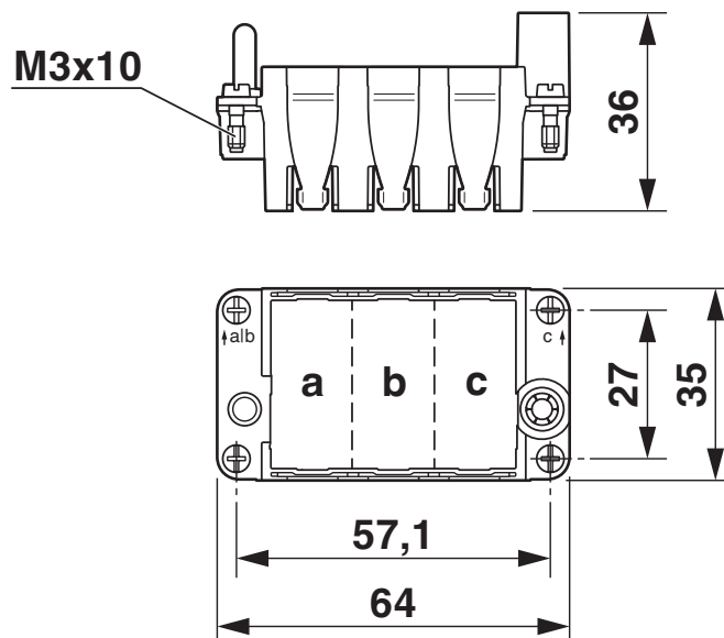
Dessin coté
