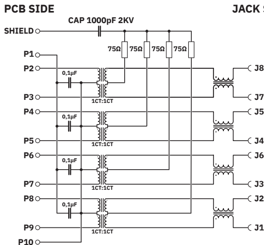
Schaltplan JACK SIDE
