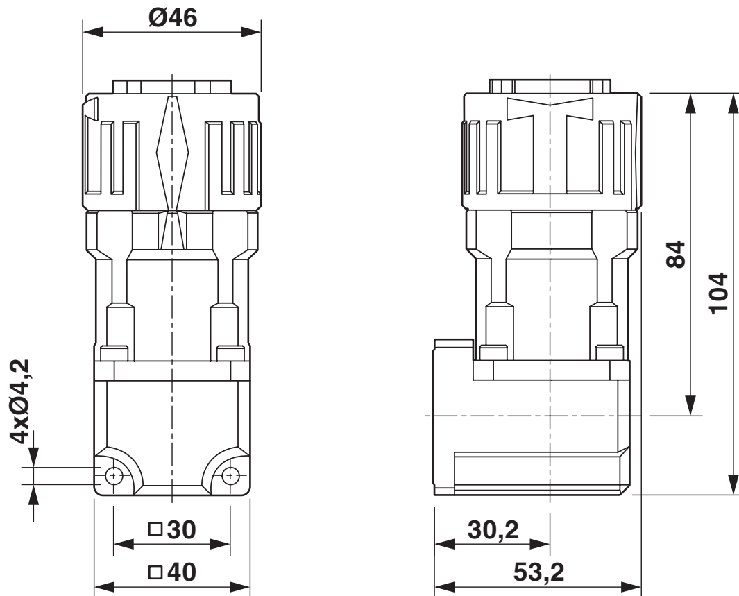
Maßzeichnung
