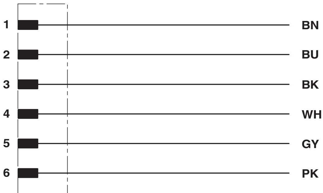
Diagrama eléctrico
