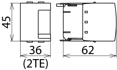
Dimensioni DSE MOD 60
