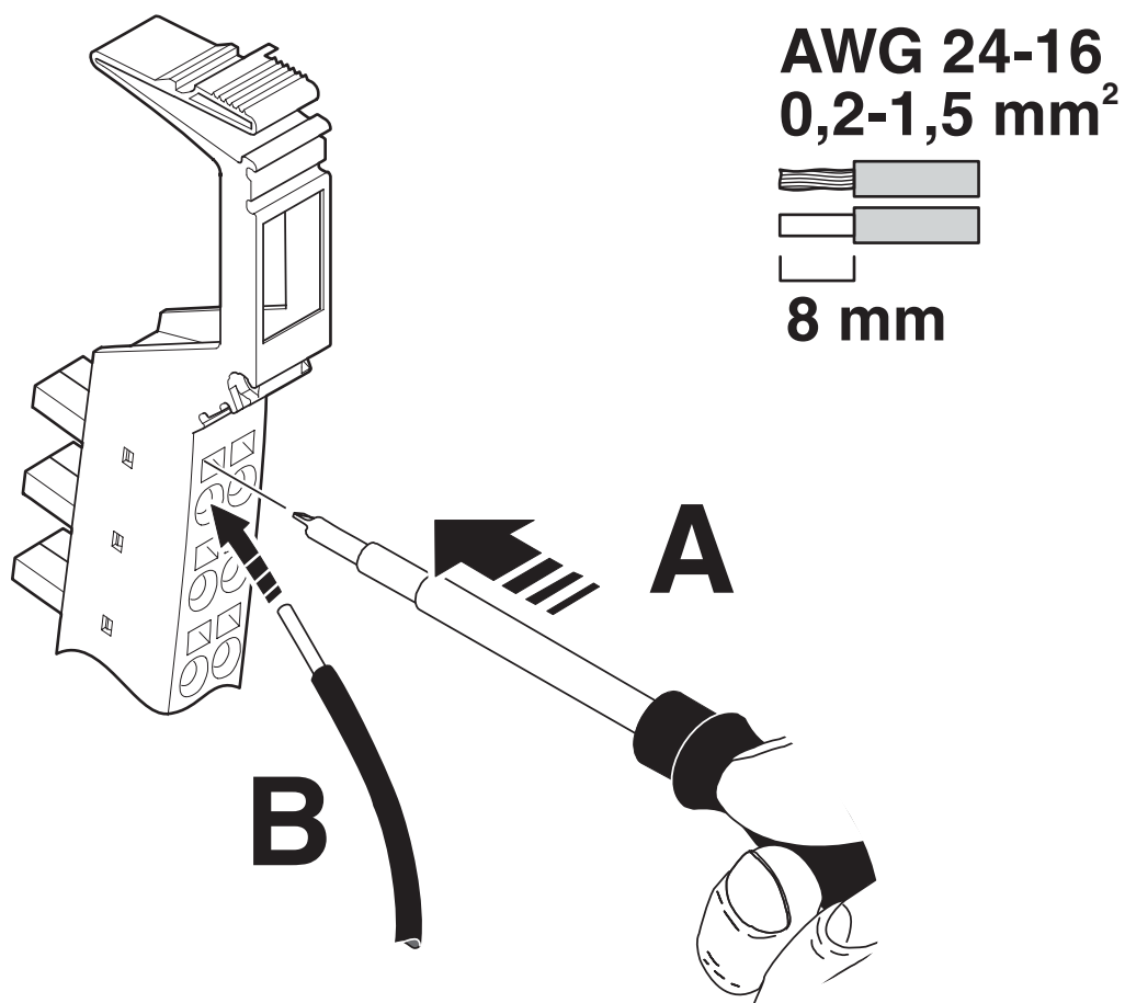
Dessin schématique
