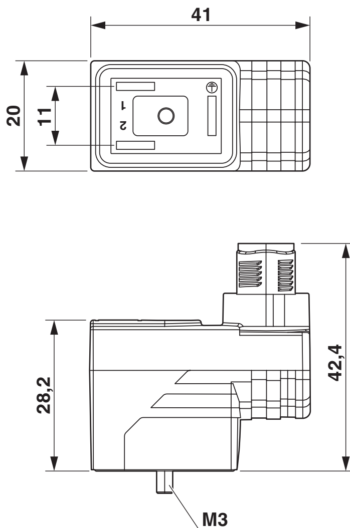
Dessin coté
