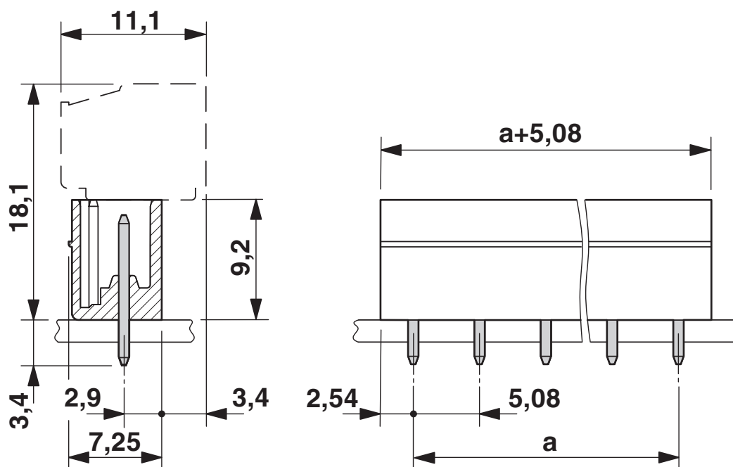
Dessin coté
