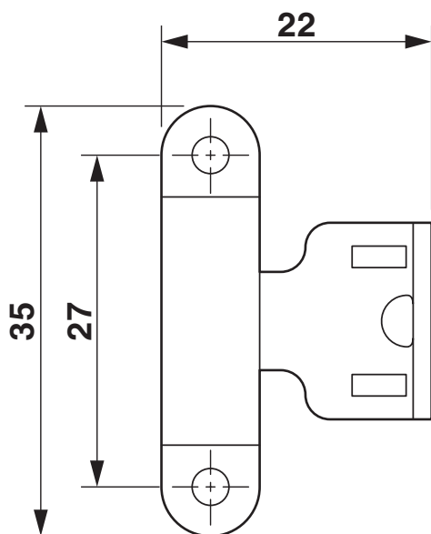
Maßzeichnung
