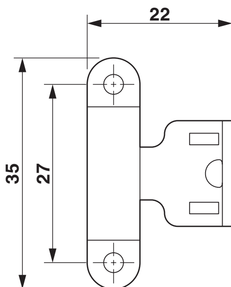
Dessin coté
