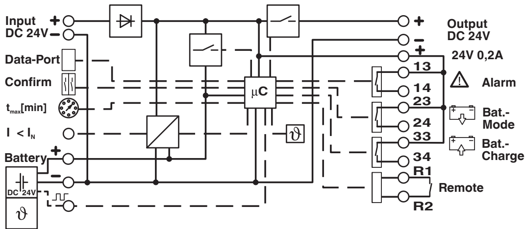
Schéma fonctionnel
