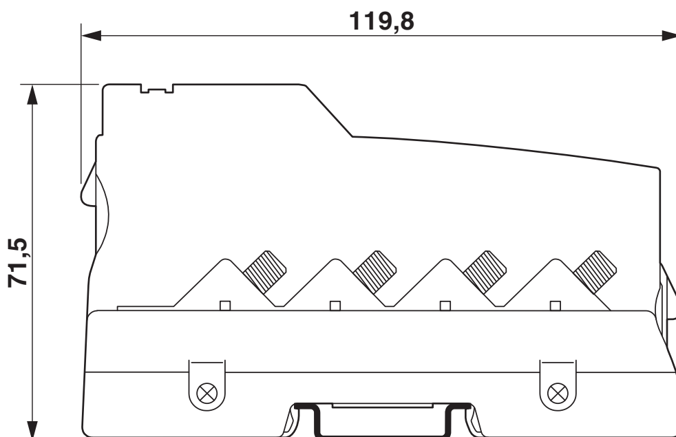
Dessin coté
