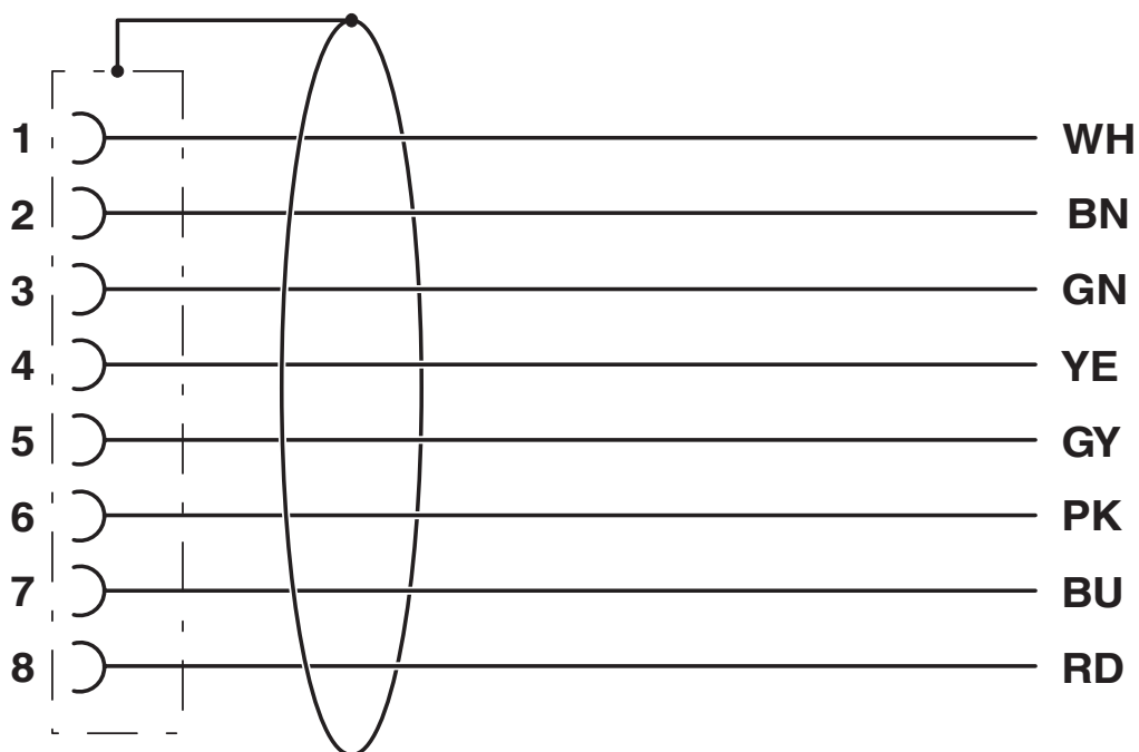
Ocupación de contactos del conector hembra M12
