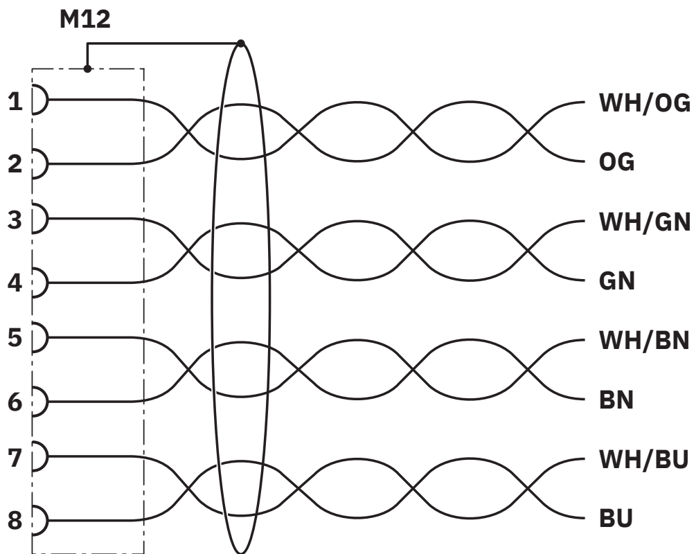
Diagrama eléctrico
