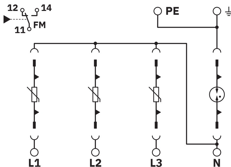
Diagrama eléctrico
