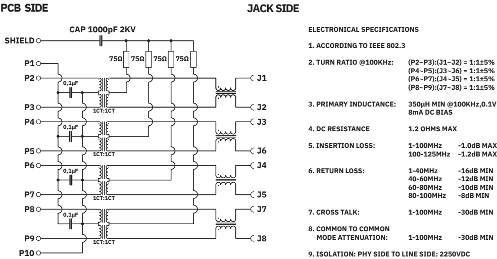
Diagrama eléctrico
