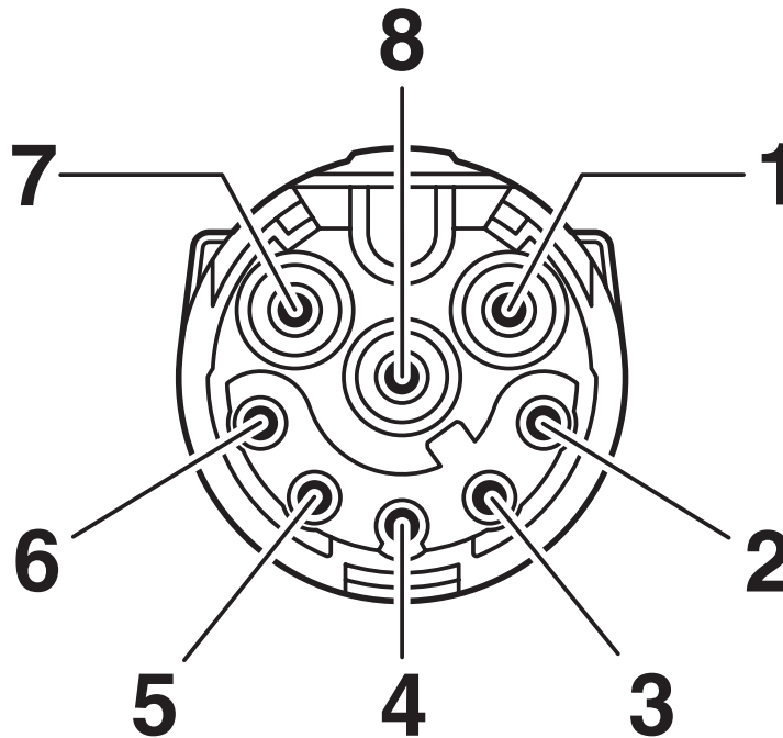
Schemazeichnung
