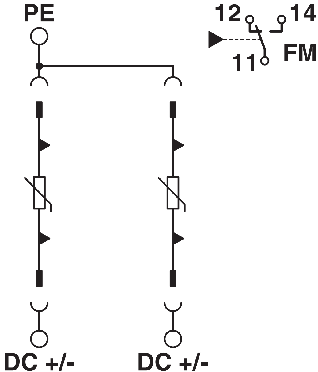
Schaltplan
