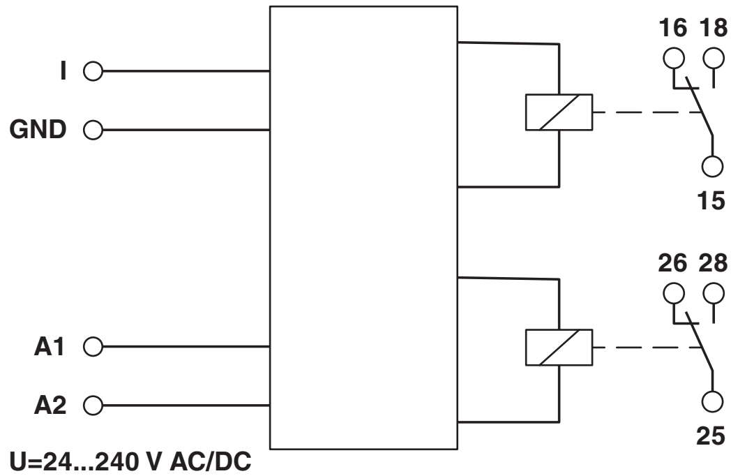
Schéma fonctionnel
