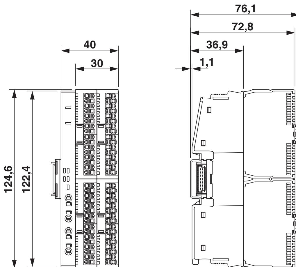
Dessin coté
