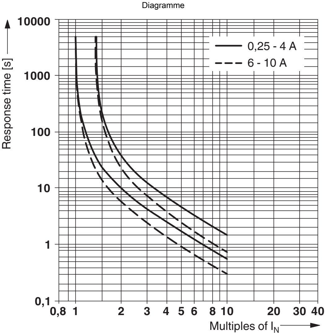
Courbe de déclenchement
