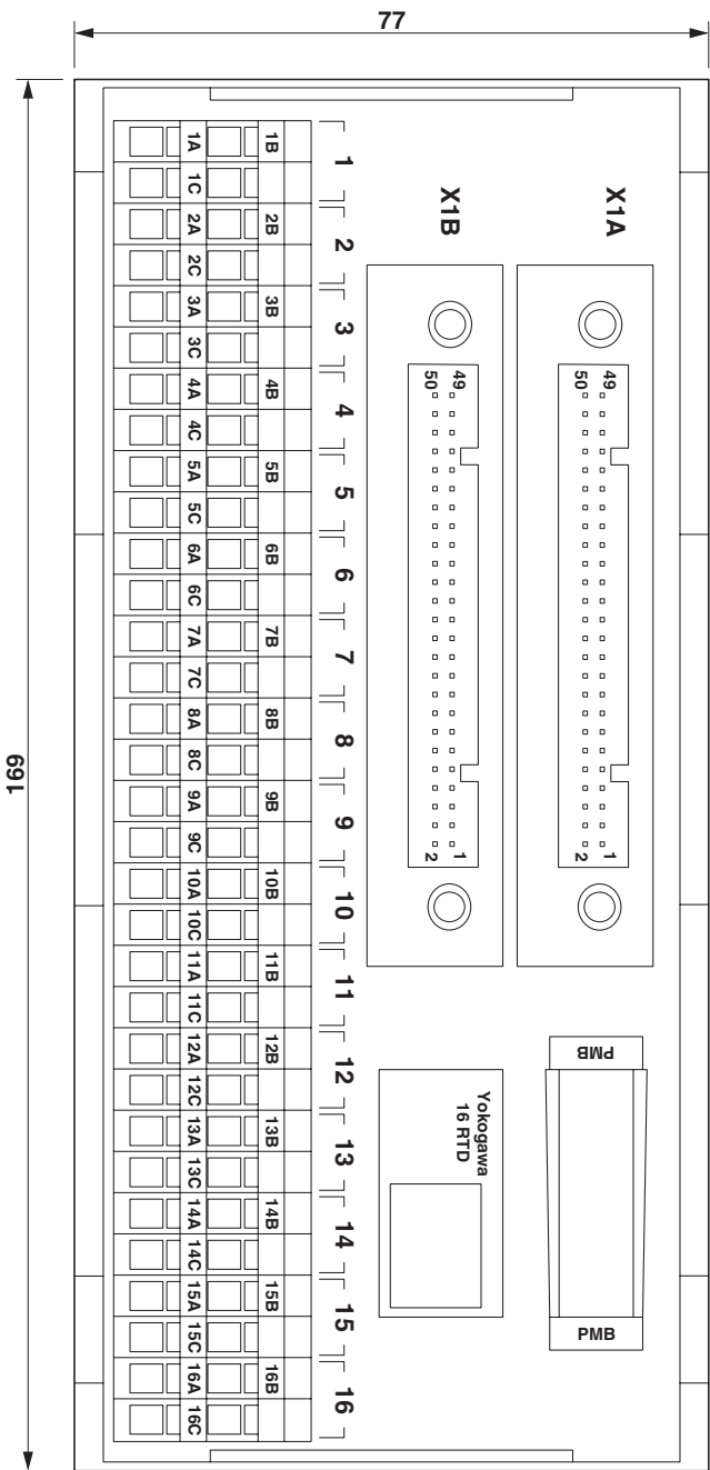
Dessin coté
