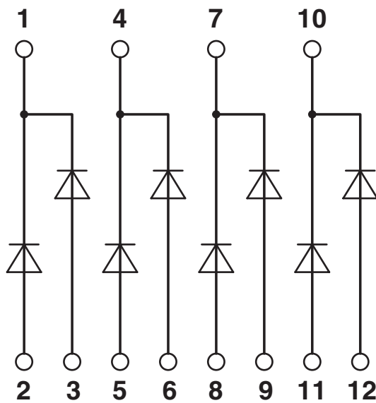
Schaltplan
