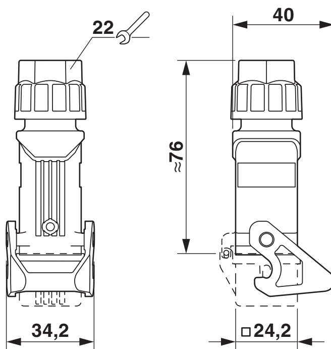
Dessin coté
