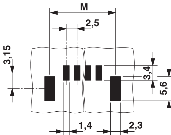
Bohrplan/Lötpadgeometrie
