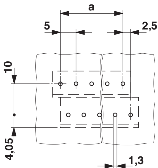
Esquema de taladros/geometría pads soldadura
