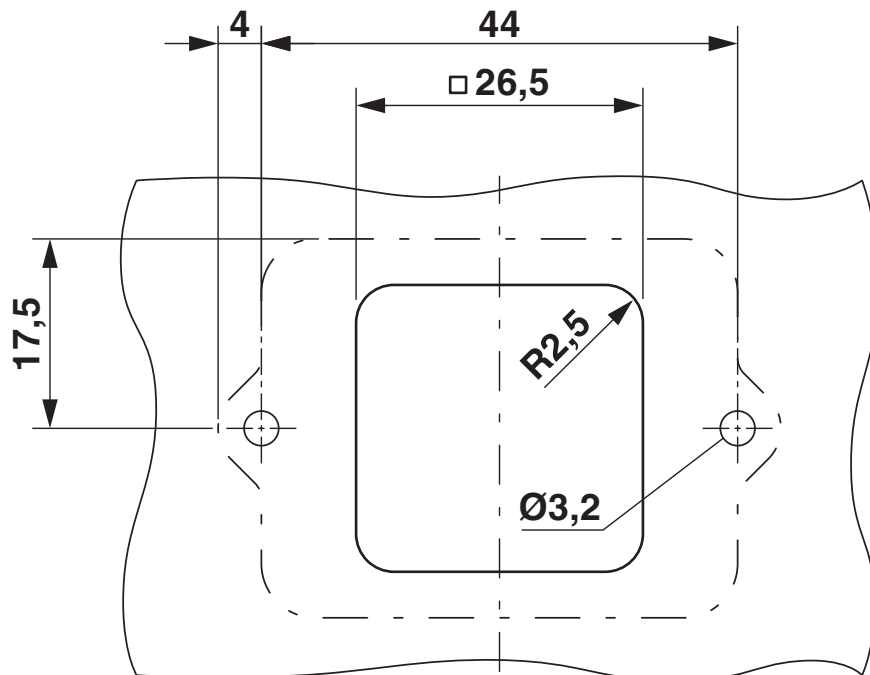
Maßzeichnung
