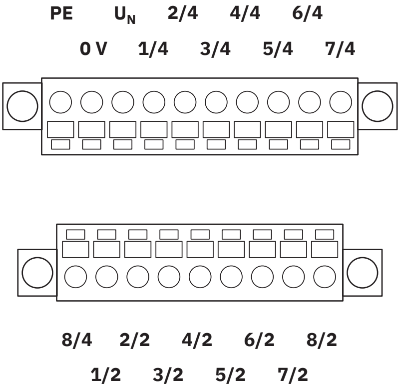
Schéma de l'affectation des broches du bloc de jonction pour C.I.
