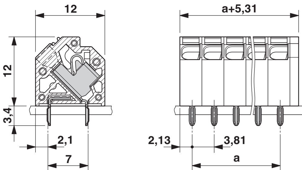
Maßzeichnung
