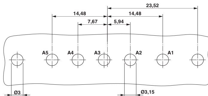
Gabarit perçage / géom. pastille soudage
