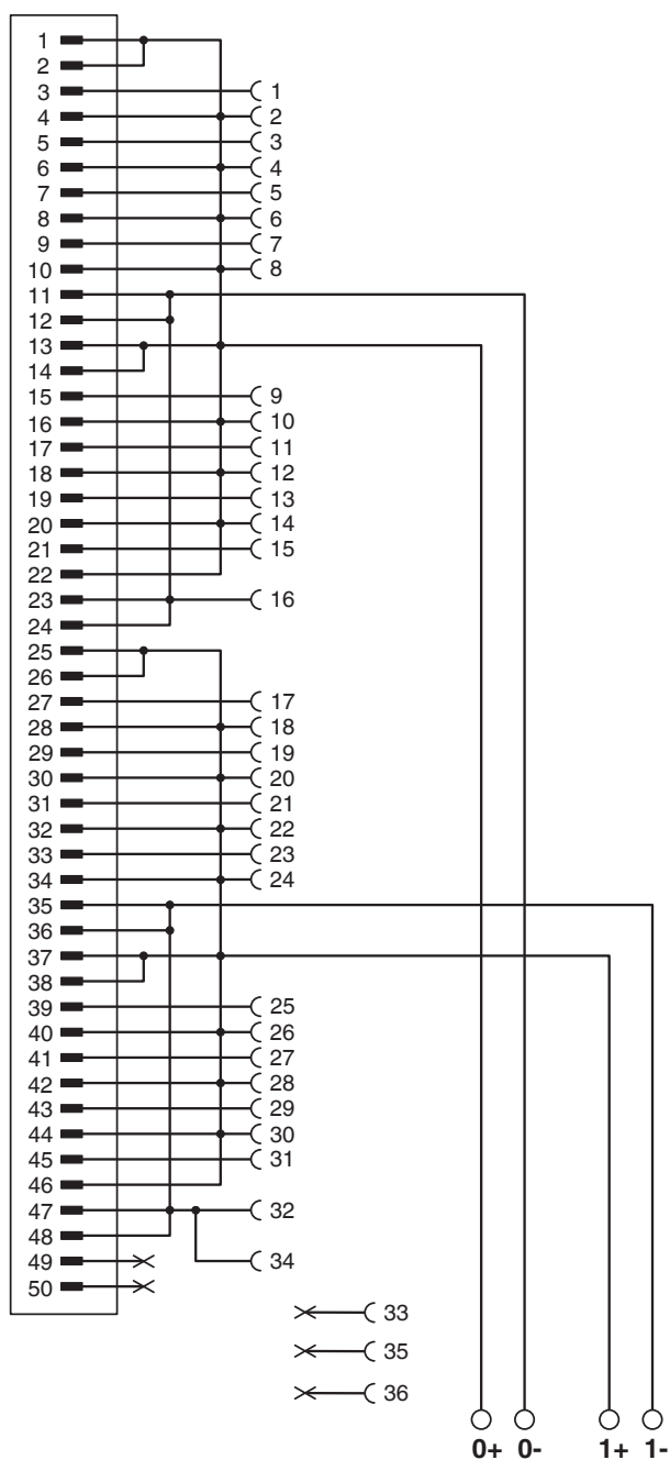
Diagrama eléctrico
