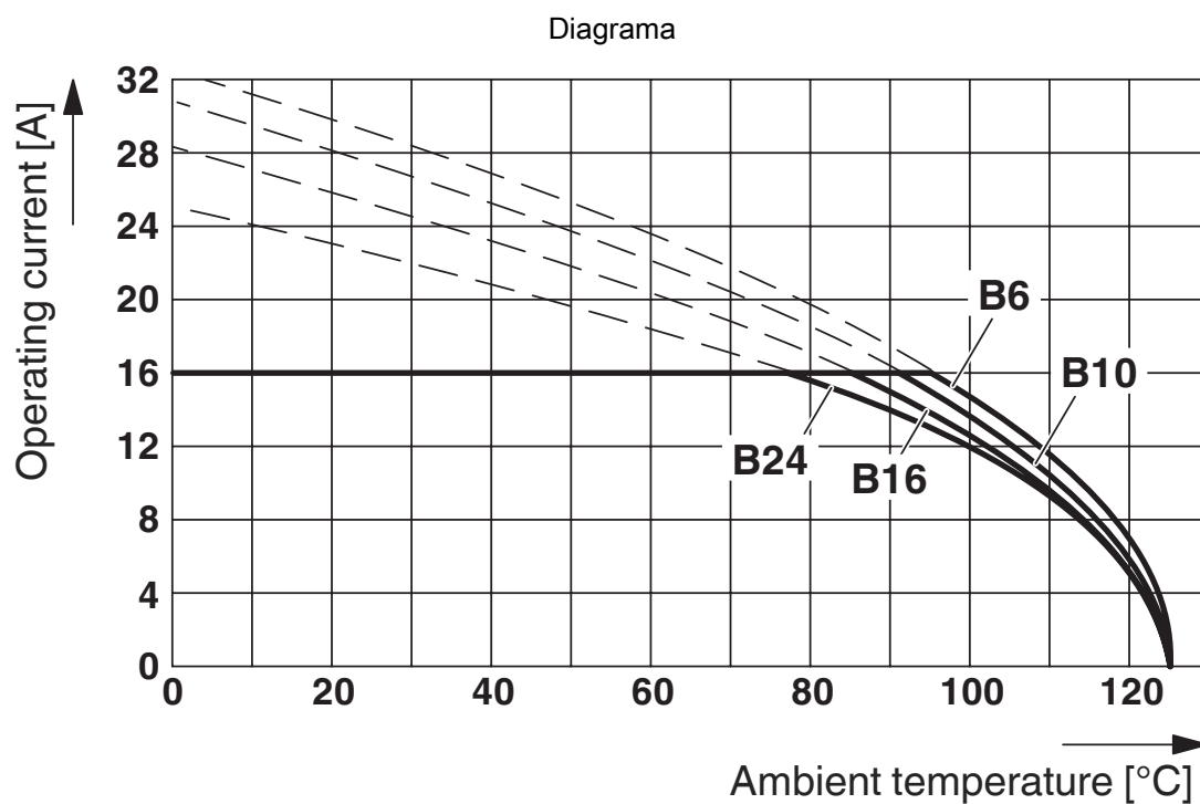
Diagrama derating, Sección de conductor 2,5 mm 2
