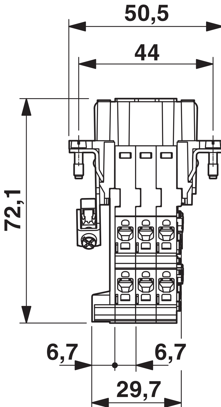
Dessin coté
