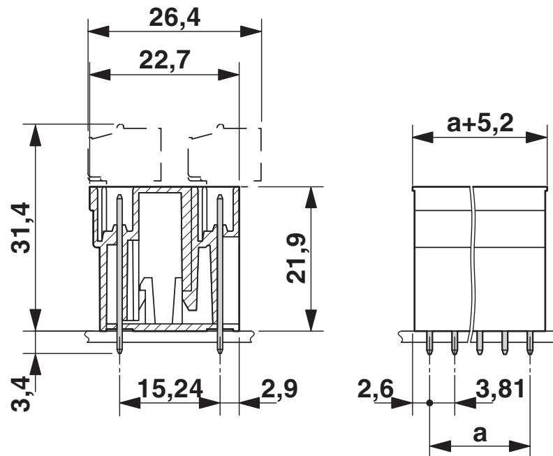
Maßzeichnung
