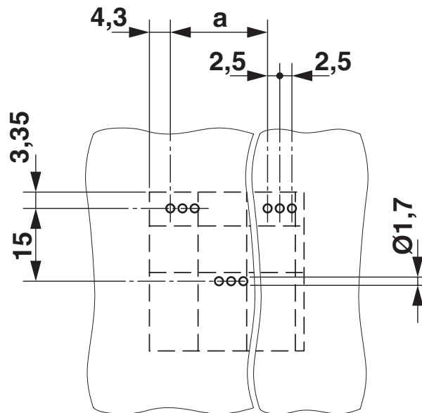
Bohrplan/Lötpadgeometrie
