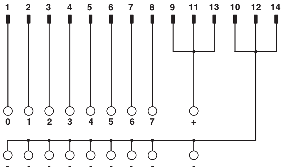
Esquema de conexiones VIP-2/.../FLK14/8M/PLC
