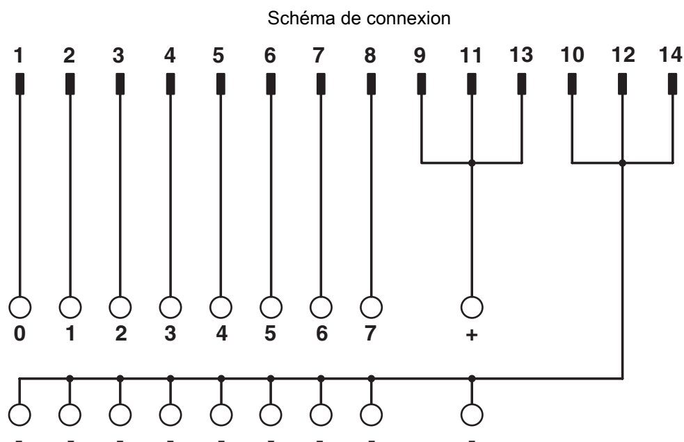
Schéma des connexions VIP-2/.../FLK14/8M/PLC
