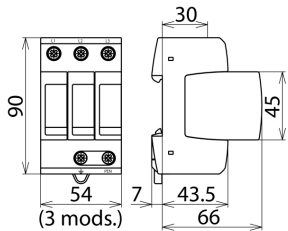
Dimensiones del DG M TNC 275
