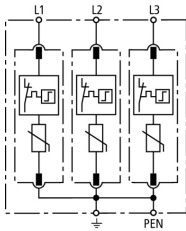
Esquema del DG M TNC 150
