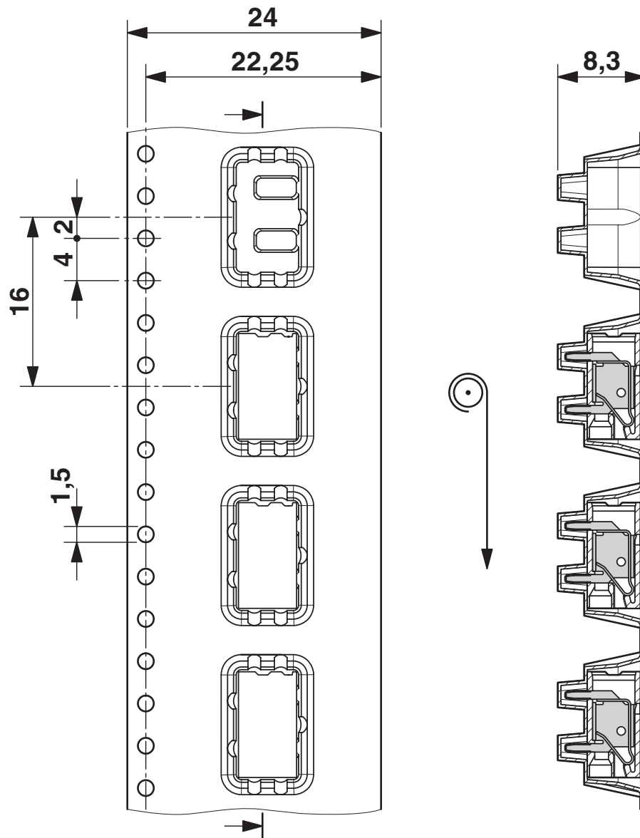
Maßzeichnung
