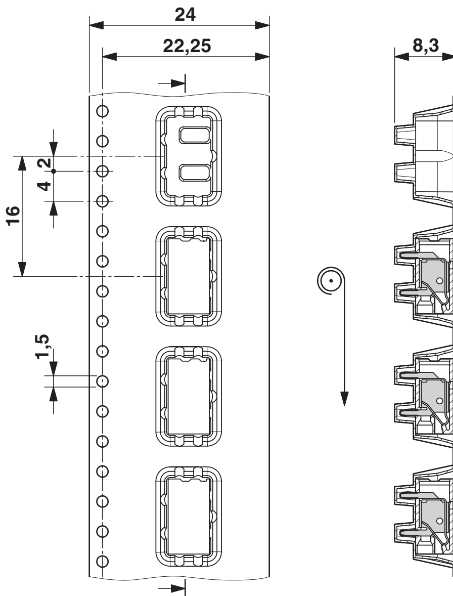
Dessin coté
