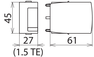
Maßbild DG MOD E H 1000 VA
