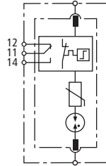
Prinzipialschaltbild DG MOD E H 1000 VA
