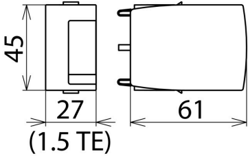
Dimensiones del DG MOD E H 1000 VA
